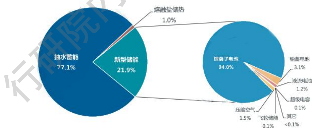
图 6 中国电力储能市场累计装机规模（2000—2022 年）
