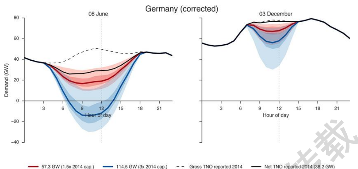
图 5 2014 年德国传统能源发电行业面临的需求曲线
